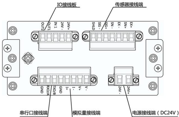
M02 后面板图
