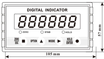
前面板尺寸(mm): 105×57
