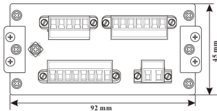
后面板尺寸(mm): 92×45
