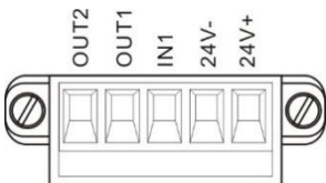
开关量端子定义图
